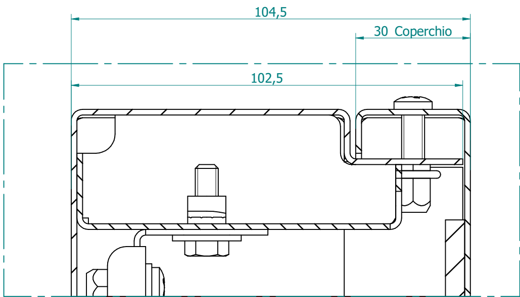
DETTAGLIO B
