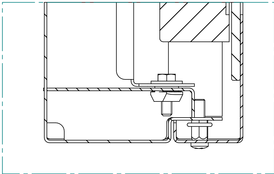
DETTAGLIO C
