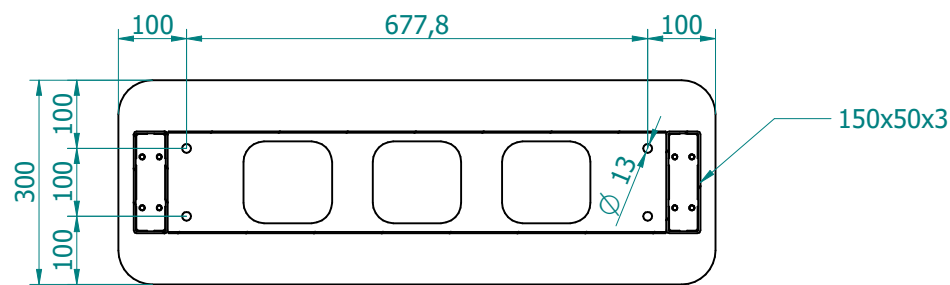
SEZIONE A-A
