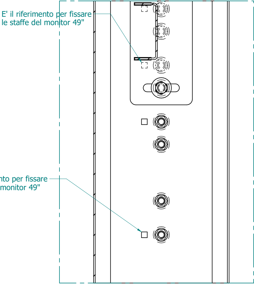
DETTAGLIO B
