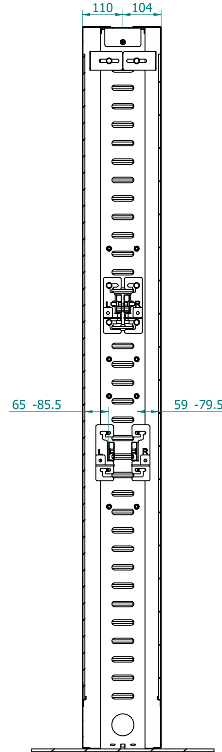
SEZIONE B-B
