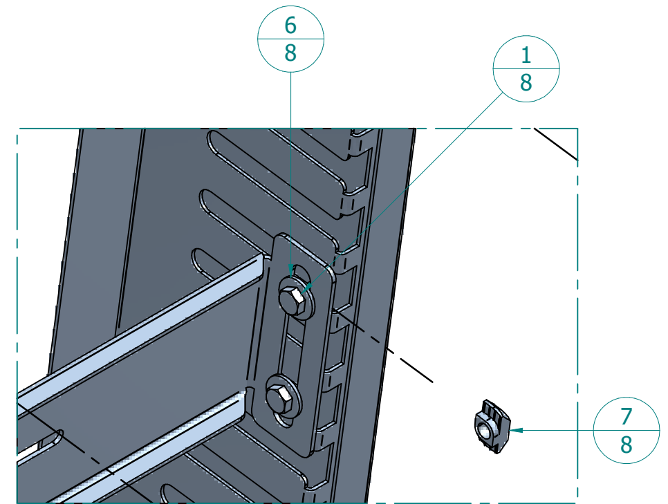
DETTAGLIO B
