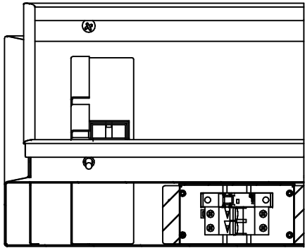
SEZIONE C-C
