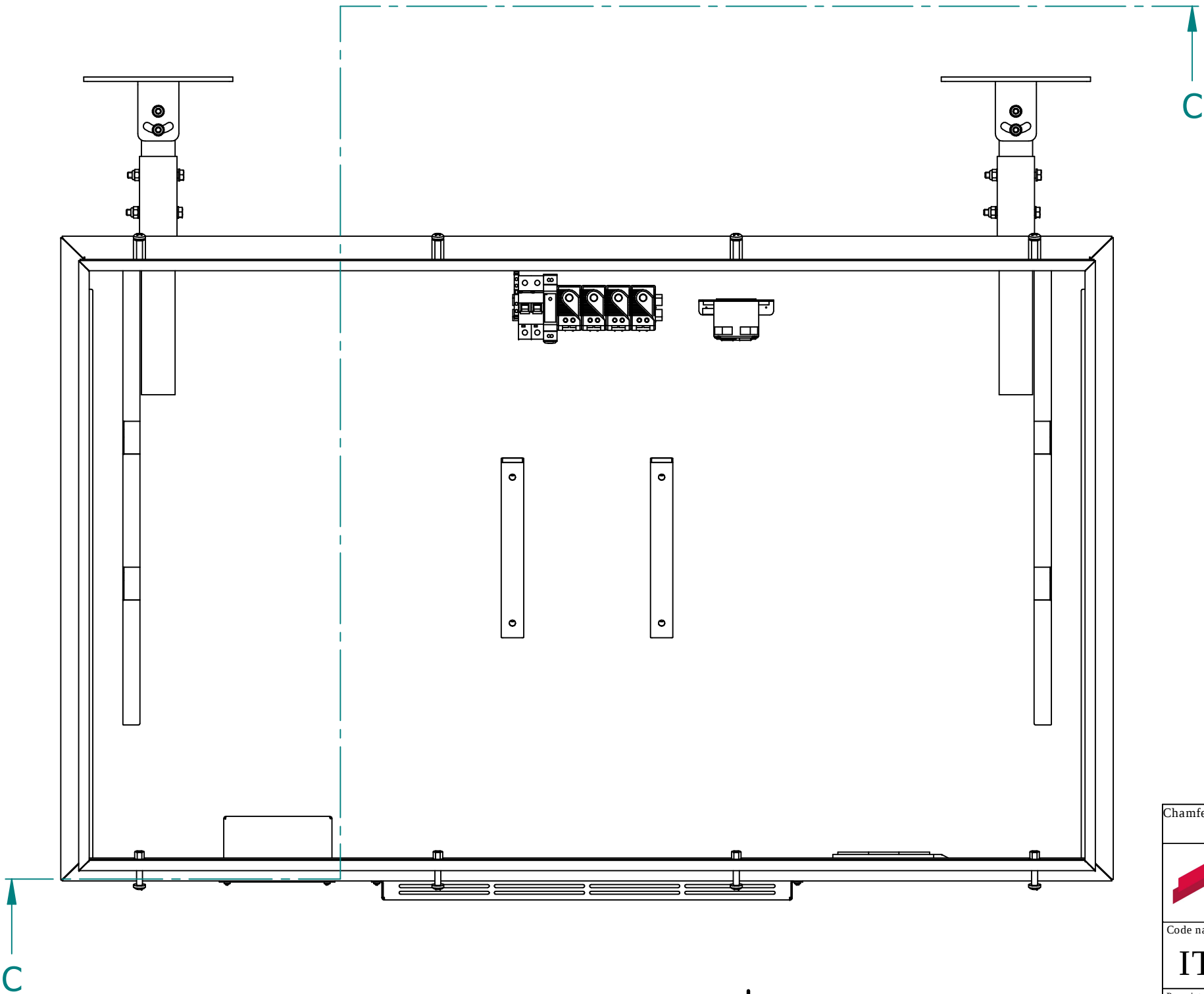
SEZIONE C-C
