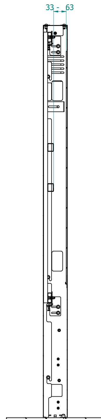
SEZIONE A-A
