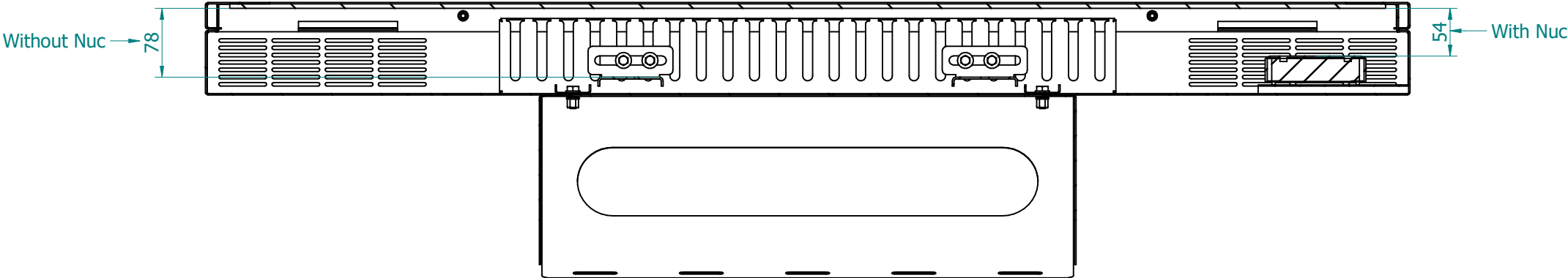
SEZIONE D-D
