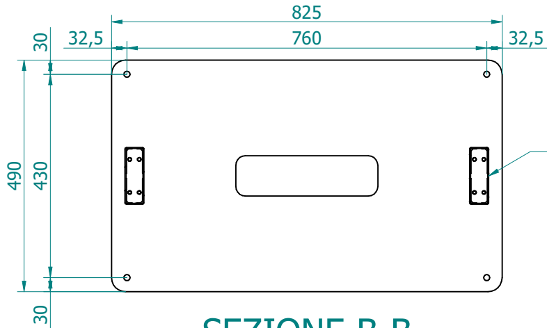
SEZIONE B-B
