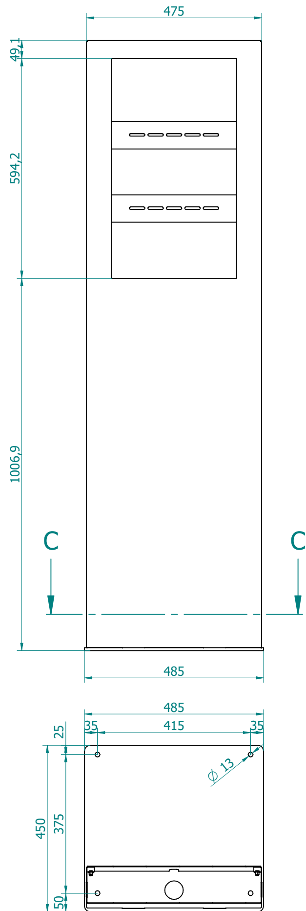
SEZIONE C-C
