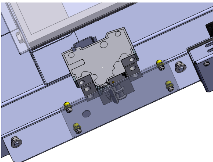
Dettaglio gruppo magnetotermico
