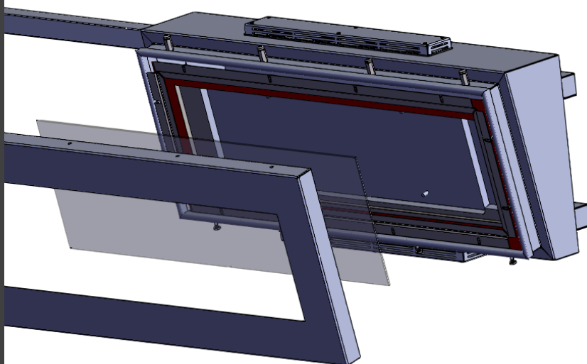
Esploso con vista cover frontale e vetro di protezione
