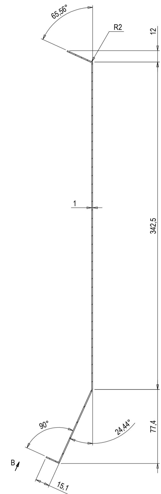
SEZIONE A-A
